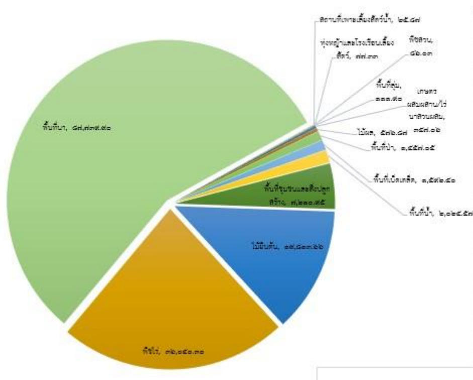
ภาพที่ ๑๔ กราฟแสดงประเภทการใช้ประโยชน์ที่ดิน อำเภอทุ่งศรีอุดม จังหวัดอุบลราชธานี
