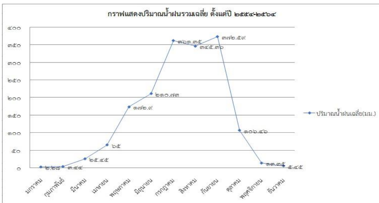
กราฟแสดงปริมาณน้ำฝนรวมเฉลี่ยตั้งแต่ปี ๒๕๕๕-๒๕๖๔
